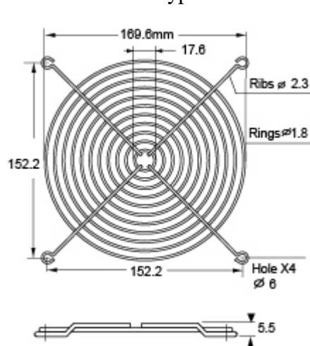
TWG-180 for 180mm Fan Standard Type
